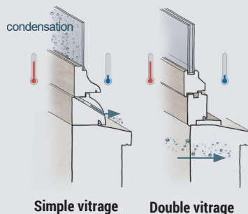
Simple vitrage
